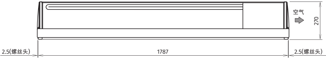
正视图
