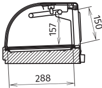
断面侧视图
