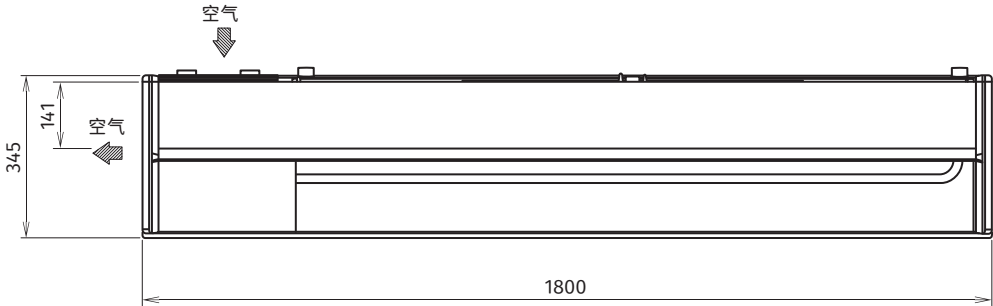
俯视图
