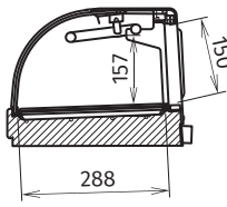
断面侧视图
