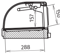
断面侧视图
