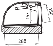
断面侧视图
