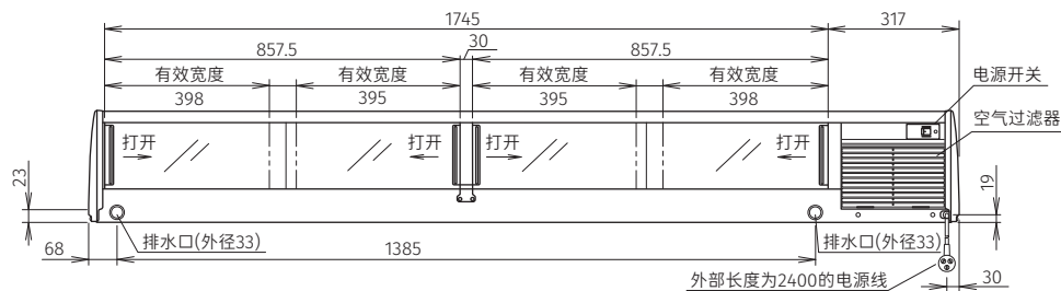
HNC-210BC-L-B
