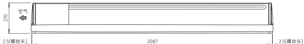
HNC-210BC-L-B
